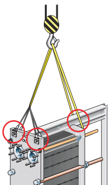
Figura 7: Elevación del modelo MK15 semisoldado.
