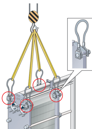
Figura 9: Elevación del modelo MA30.
