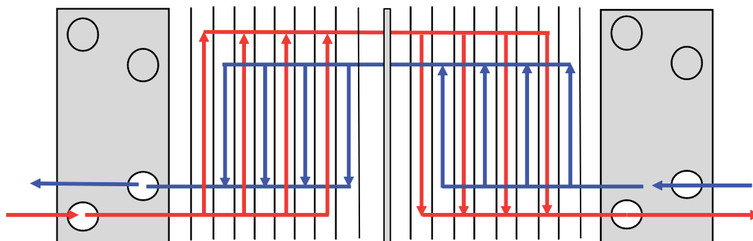
Figura 3: Ejemplo de una configuración de múltiples pasos.
