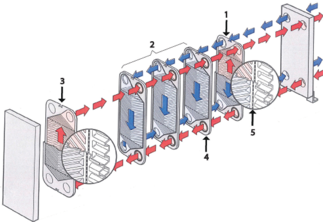
Figura 2: Ejemplo de una configuración de paso único.
