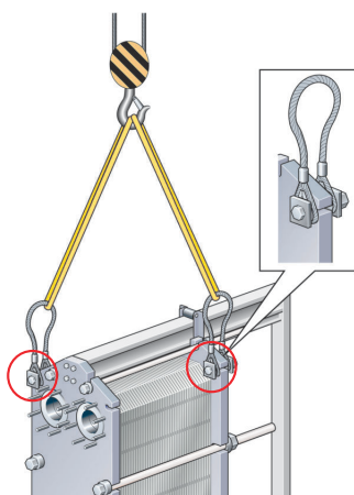
Figura 8: Elevación de los modelos TK20 semisoldado y T20 semisoldado.
