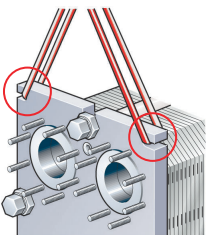
Figura 5: Elevación de los modelos M6, M10 y T10.
