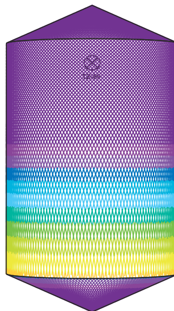
D2 H3, TZ-89 4 x Ø4 mm, time 11.1 min
